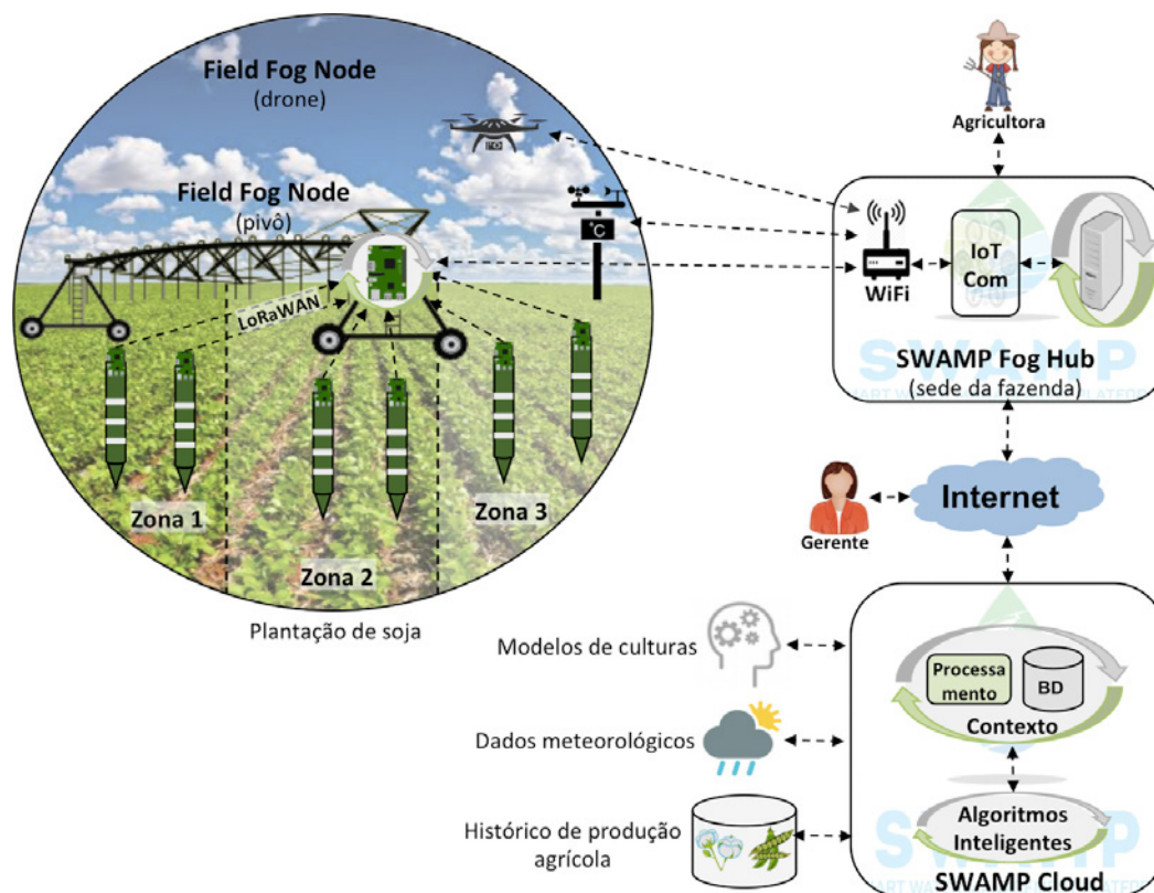
Figura 7 – Irrigação baseada em pivô central em Matopiba
